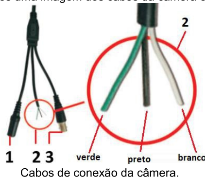
Cabos de conexão da câmera.
